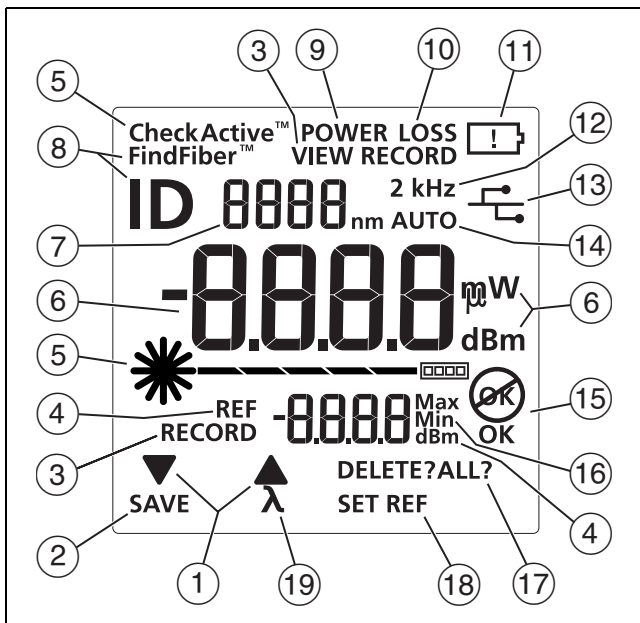
图 3. 显示屏功能
