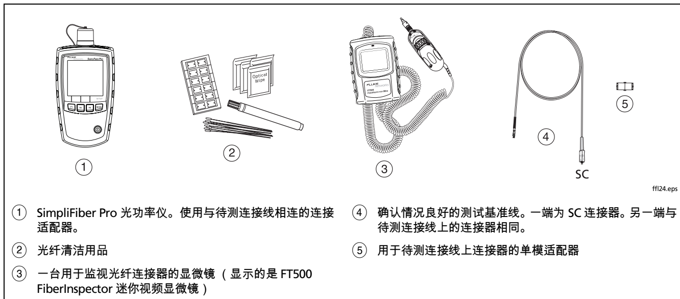
图 A-1. 用于测试测试基准线的装置
