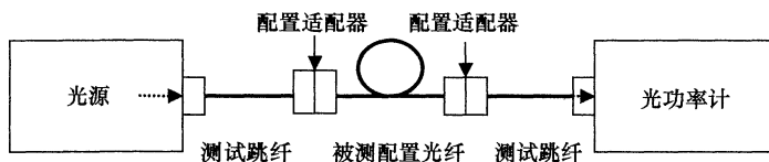
图 8 三跳线信道测试连接方式
